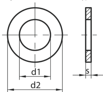
Rysunek 23 Podkładka typu M
