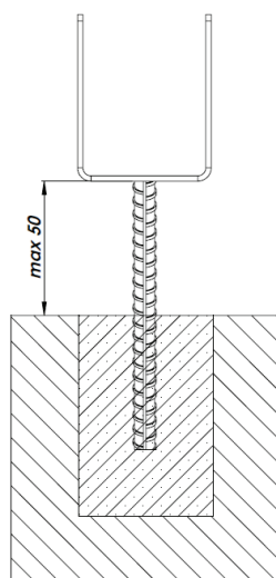
Rysunek 1 Podstawa słupa z prętem gwintowanym
