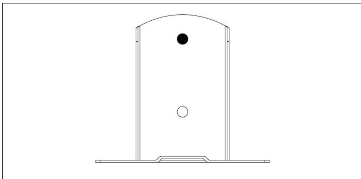
Rysunek 47 Typ PSD 90, PSD 100, PSD 120, PSD 140, PSD 160, PSD 200
