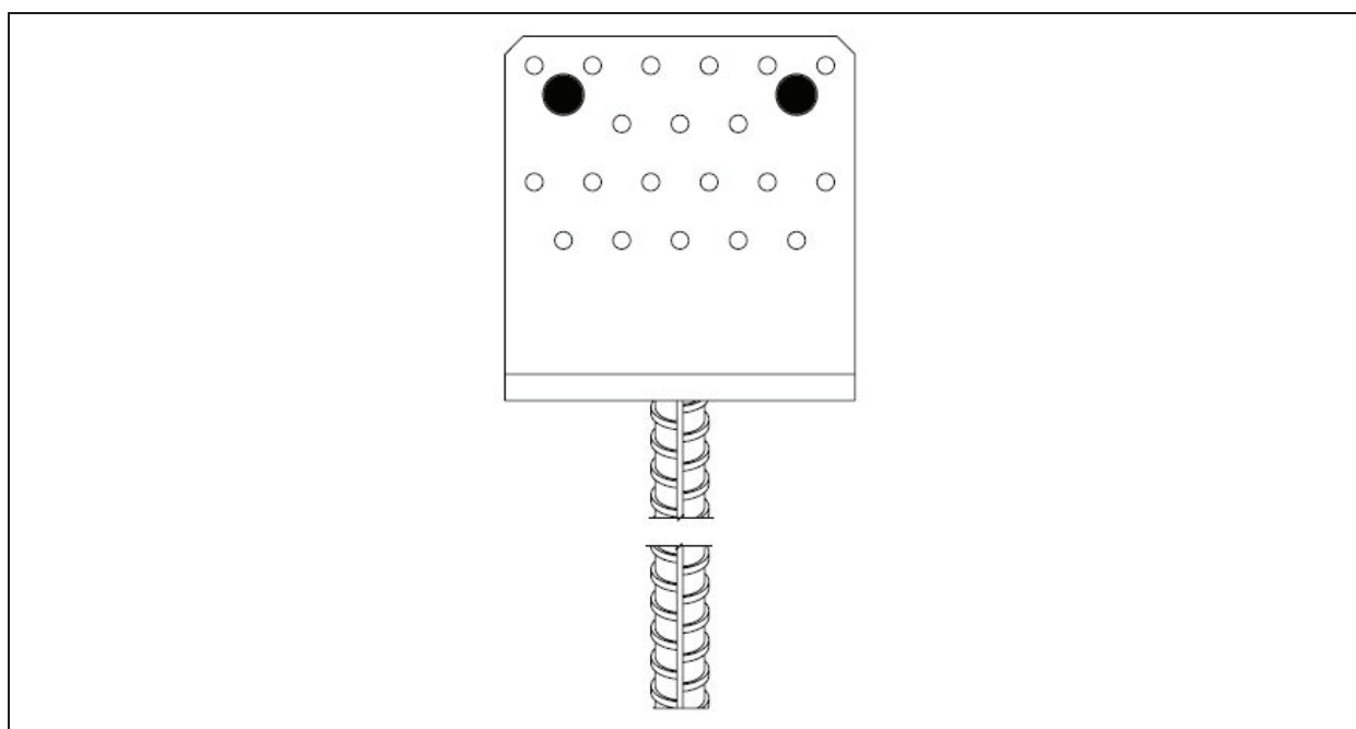
Rysunek 59 Typ PSS 100, PSS 120, PSS 140
