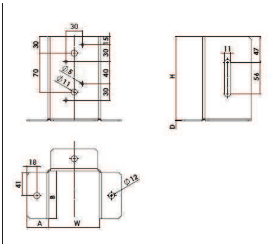
Rysunek 10 Typ PSP DX 90
