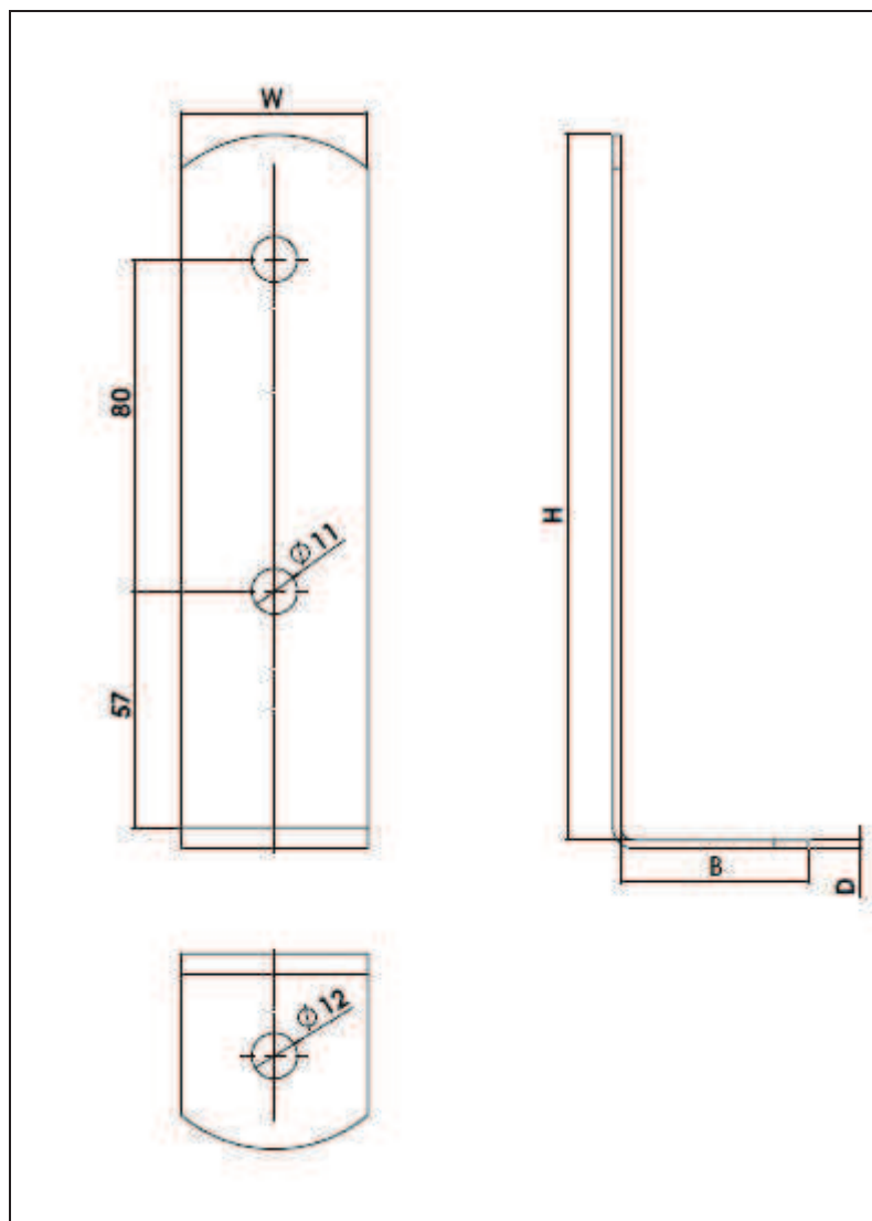
Rysunek 16 Typ PSC 45
