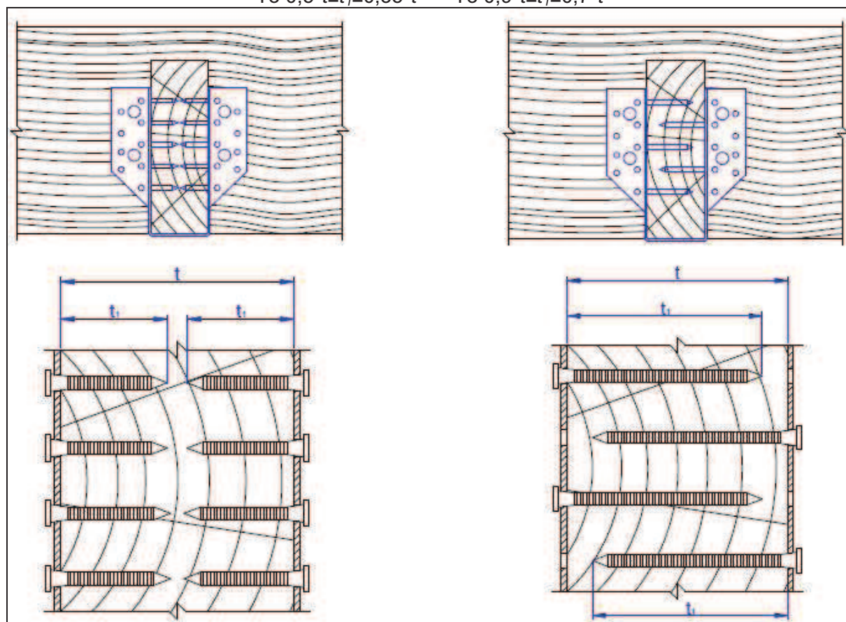
Rysunek 43 Zasada umieszczania gwoździ
