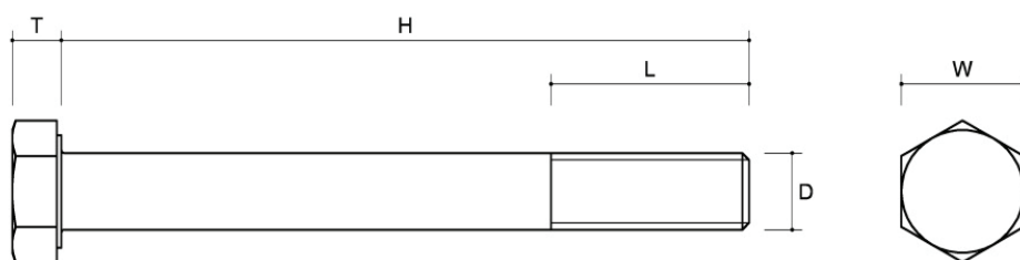
Rysunek 22 Śruba typu M
